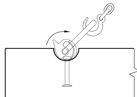
obr. 1. Nasazení zdviháku.
