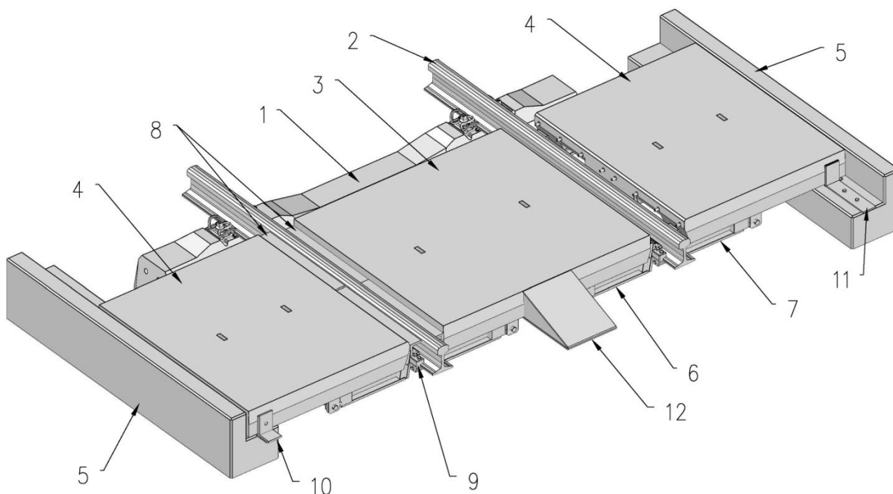
Obrázek 1 Pohled na přejezd BRENS
