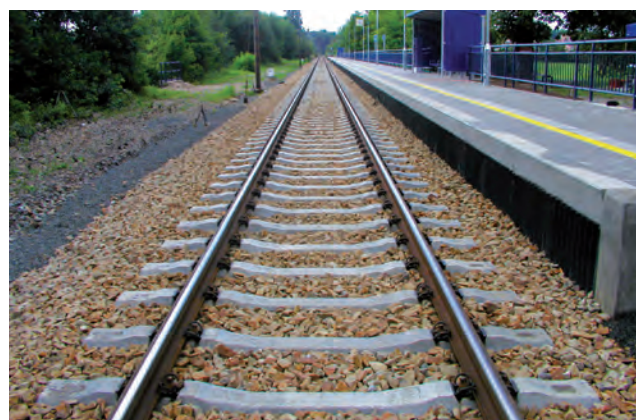
žst. Štáhlavy železobetonové pražce B 91 S, nástupištní hrany H 130 uč. protihlukové tuárnice
