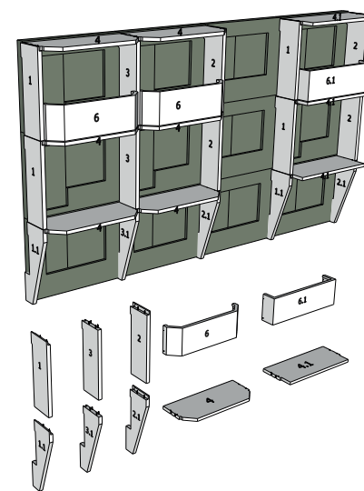
Lodžie založené na konzolové stěně patrové
