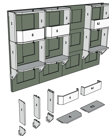
Lodžie založené na konzolové stěně krátké
