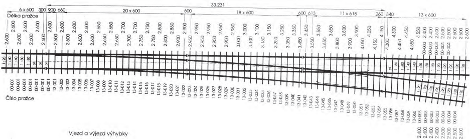
Skladba pražců výhybky UIC 60 1 : 9 - 300
