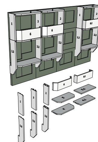
Lodžie založené na konzolové stěně dlouhé
